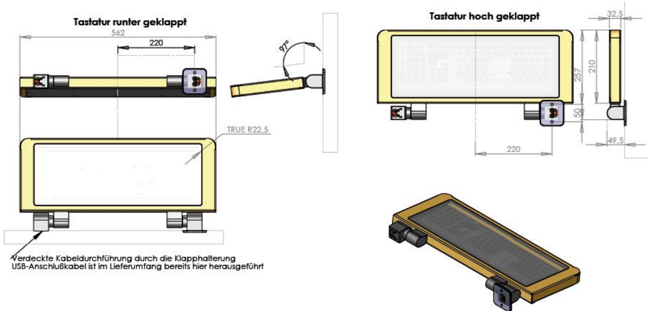
Abbildung zeigt Sonderausstattung: Wandadapter für Verschraubung von vorne
