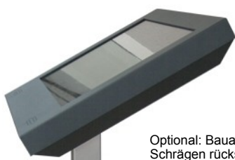
Staubdichtes Gehäuse mit von außen zugänglichen Staubfiltern
